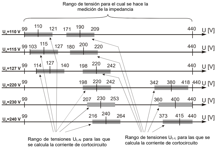
Fig. 4.6 Rangos de tensión de medición
