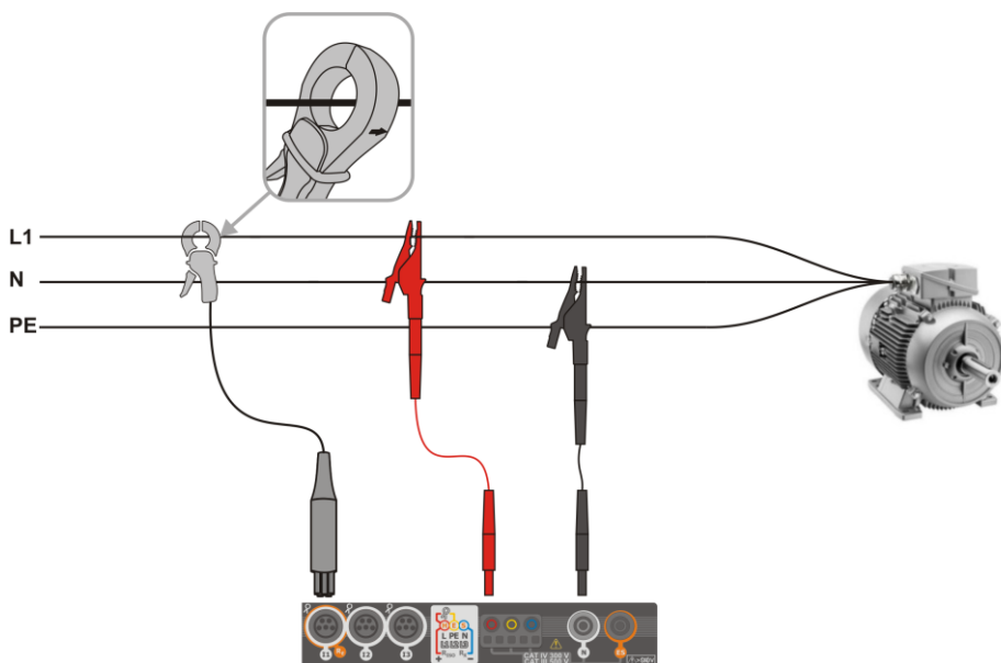
Fig. 6.4 Esquema de conexión – sistema monofásico
