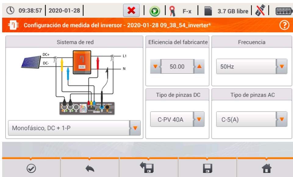
Fig. 4.10. Pantalla de configuración de la medición de la eficiencia del inversor
