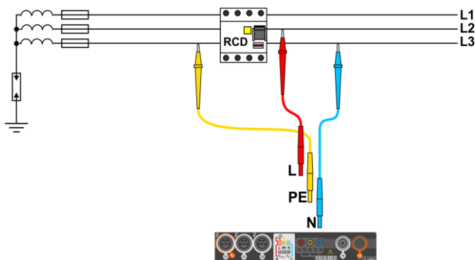
Fig. 4.9 Test del RCD y sin la participación del conductor PE
