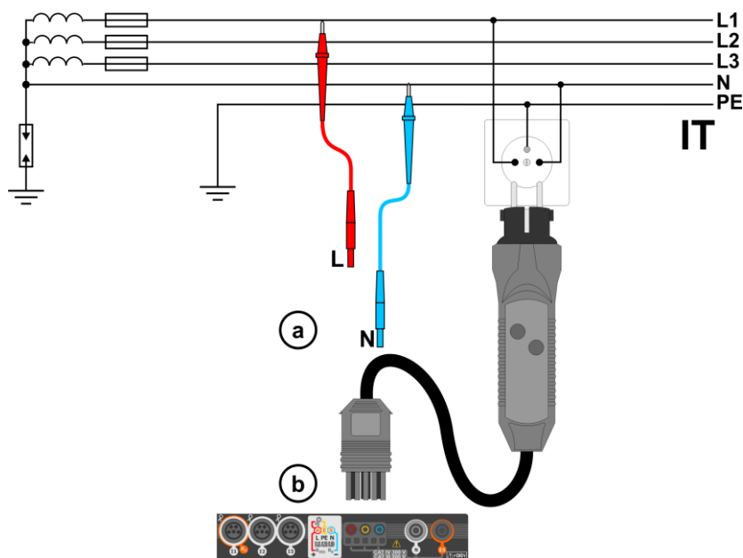
Fig. 4.7 Medición en el sistema IT
