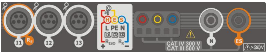
Fig. 6.1 Entradas de medición
