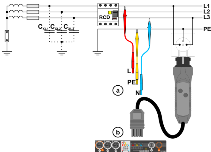
Fig. 4.8 Medición de RCD en la red IT. El circuito está cerrado por las capacidades parásitas C_x
