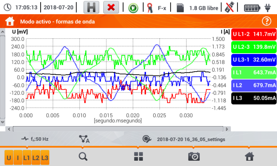
Fig. 6.13. Lecturas actuales – formas de onda
