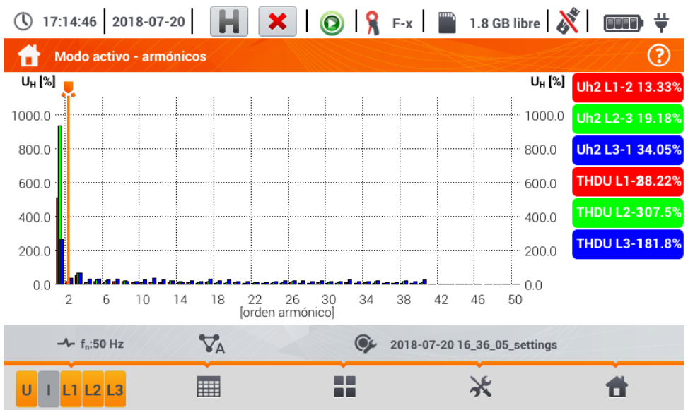
Fig. 6.17 Lecturas actuales – armónicos – vista de barras.
