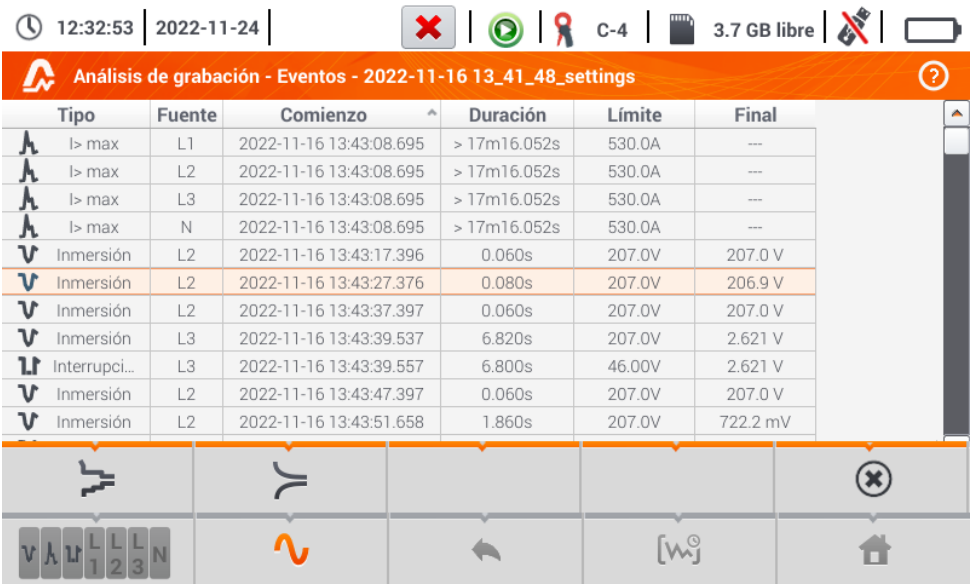
Fig. 6.25. Análisis de registro – lista de eventos
