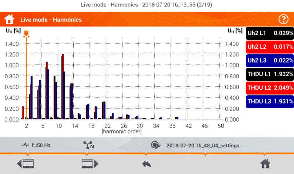
Fig. 6.12 Ejemplo de vista previa de la captura de pantalla
