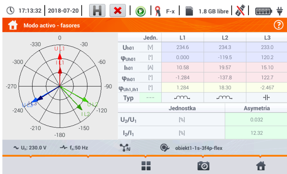
Fig. 6.16. Lecturas actuales – gráfico de fasores
